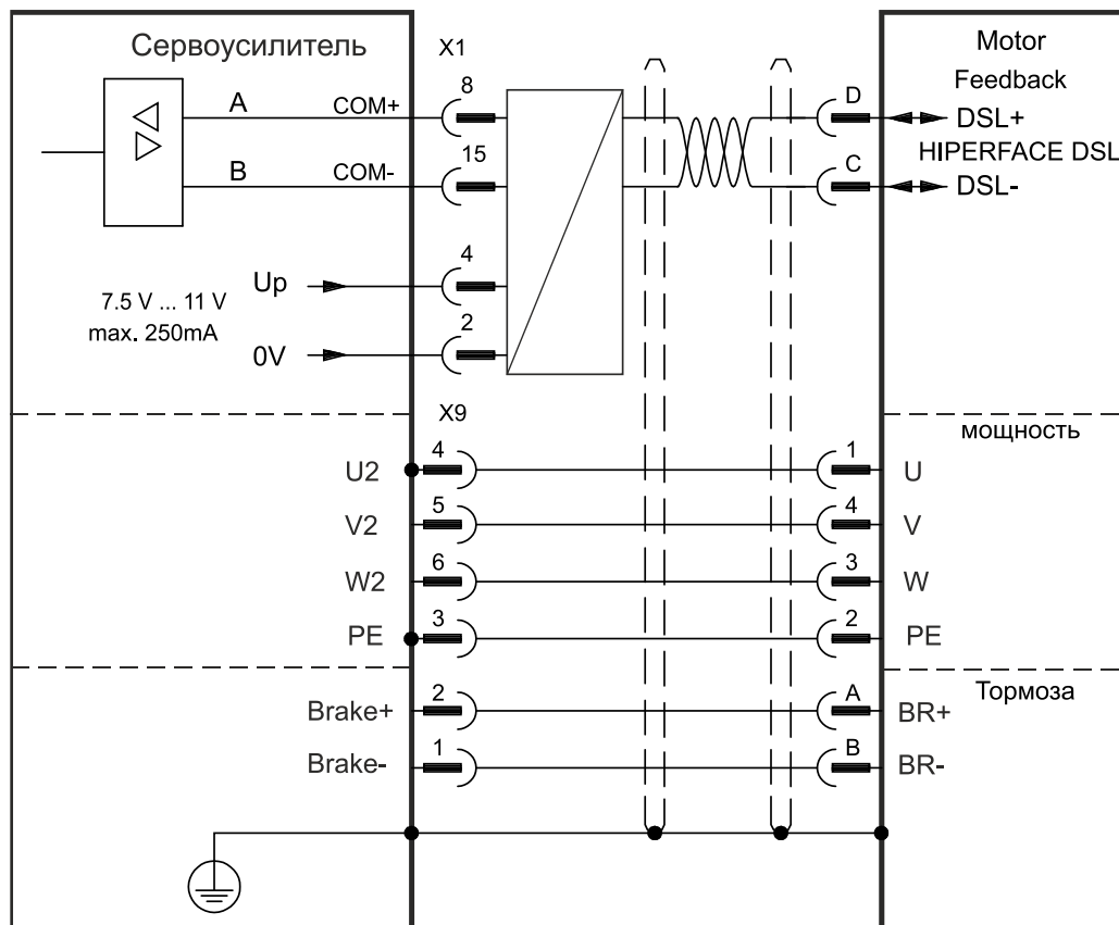
Расположение выводов со стороны датчика относится к двигателям Kollmorgen.
