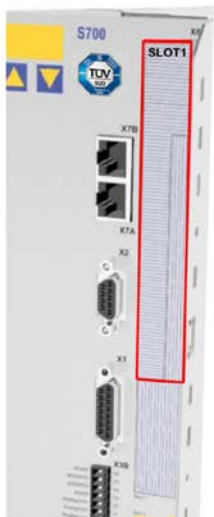
1 – Граница гнезда 1
