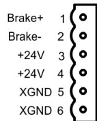
X4 24V/Brake
