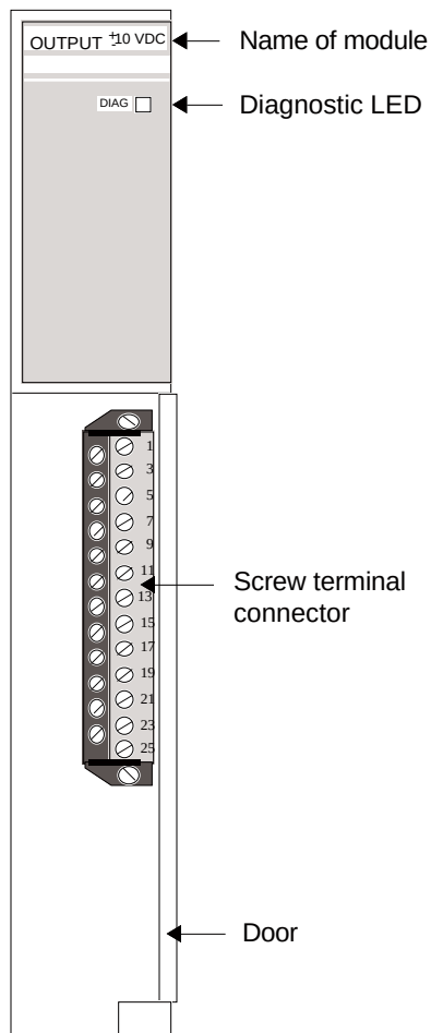
Figure E4-1. OUTPUT \pm 10\text{V} DC Module
