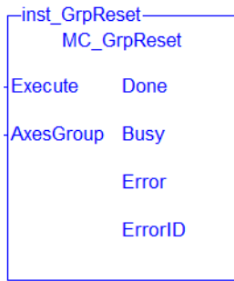
Figure 1-97: MC_GrpReset
