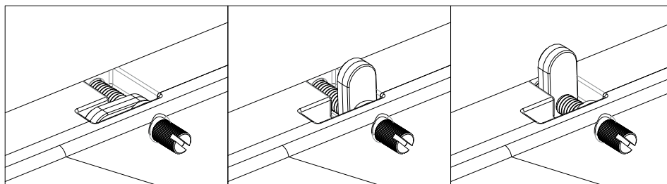
Figura 3-1: Apriete los tornillos con un par de 0,7 \text{ Nm} \pm 0,2 \text{ Nm} .
