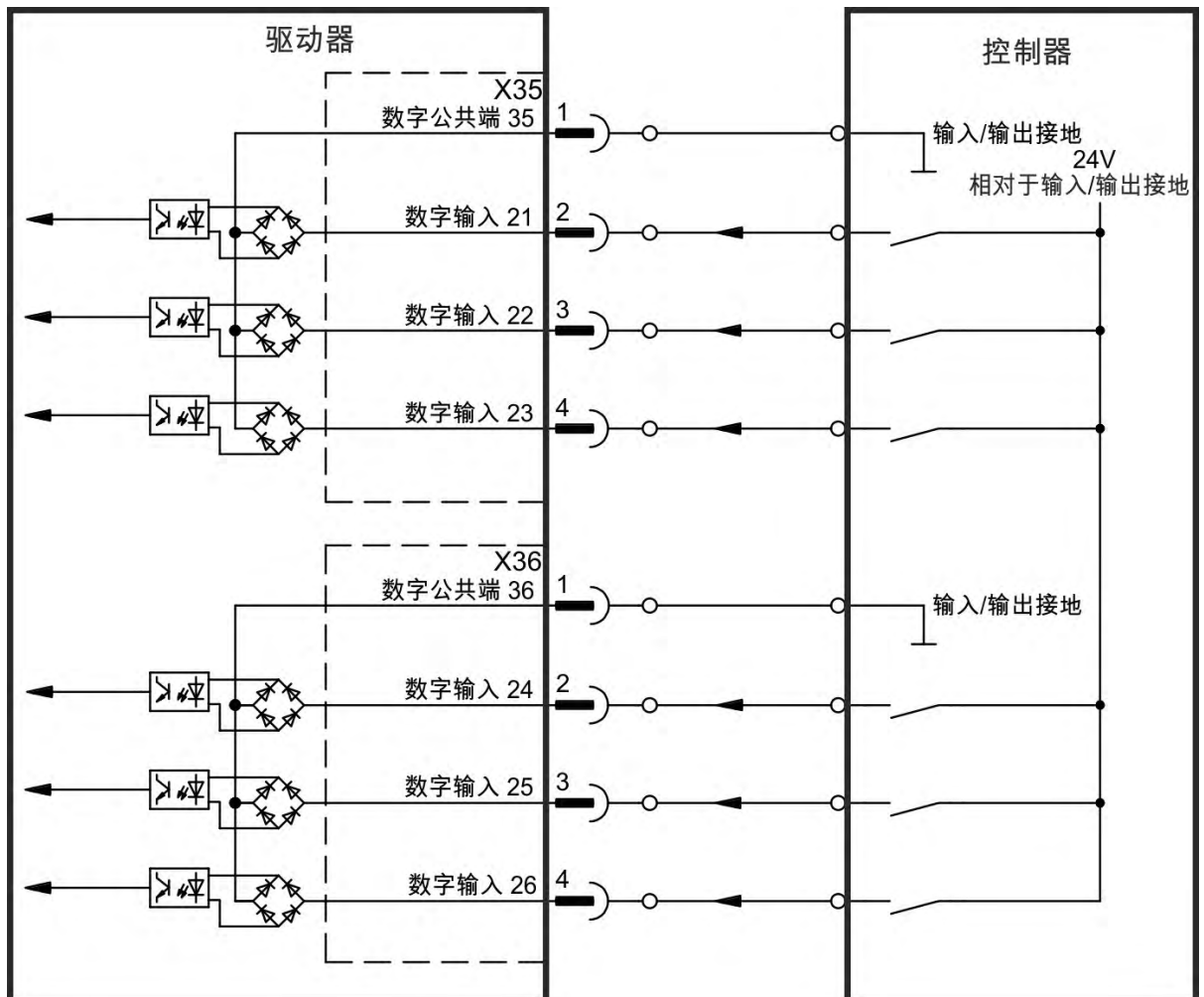
数字输入接线图(例如, 源类型连接)
