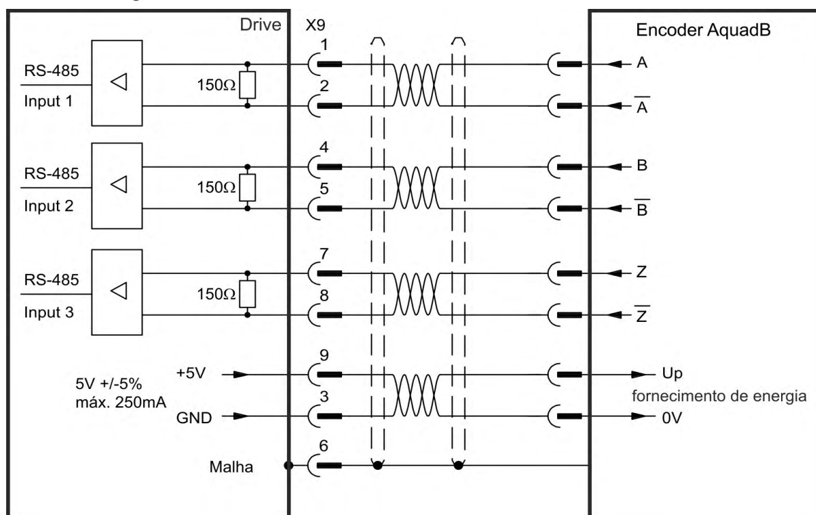
Diagrama de conexão
