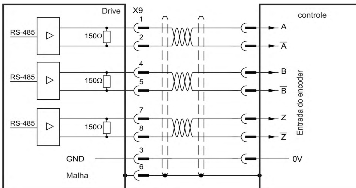
Diagrama de conexão
