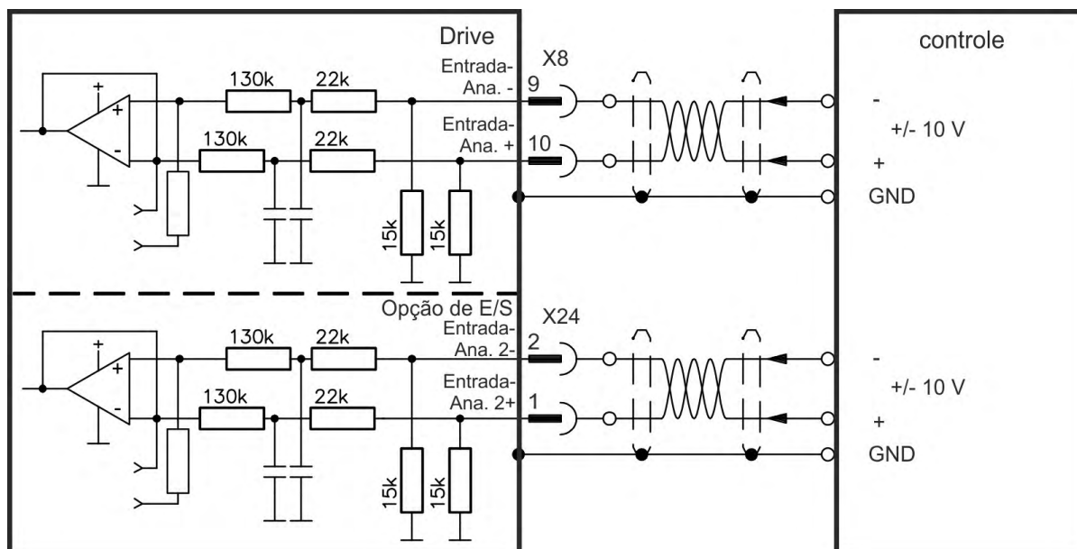
Diagrama de fiação da entrada analógica
