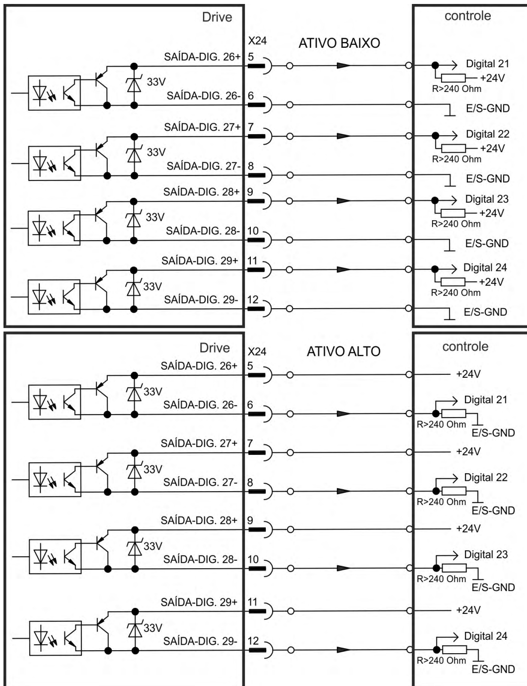
Diagrama de fiação X24
