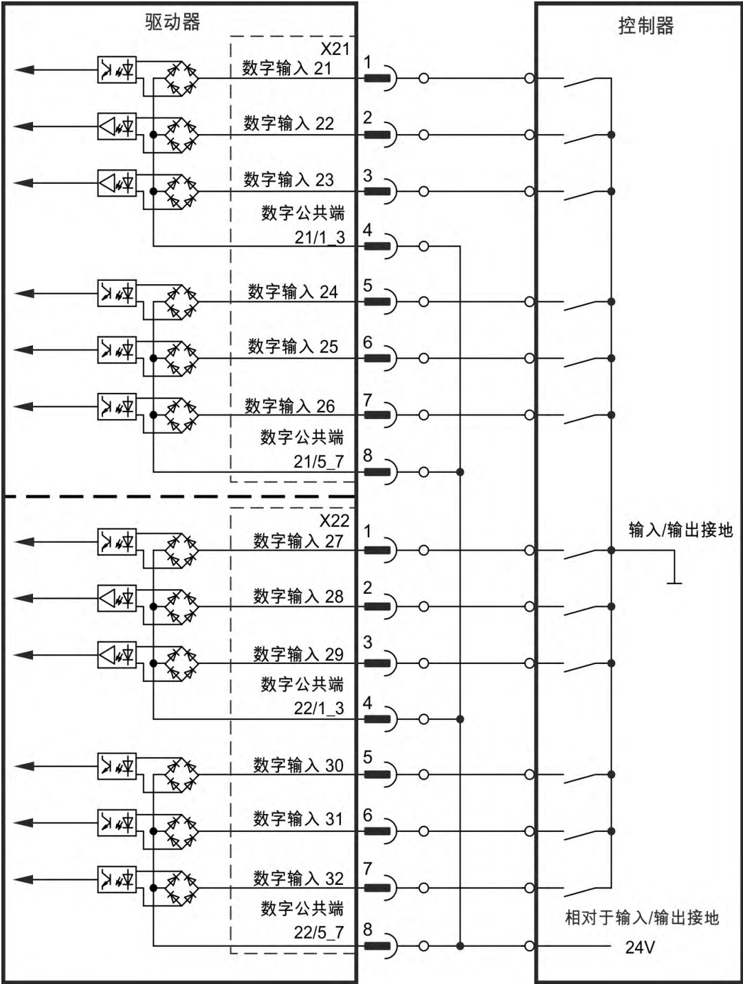
数字输入接线图(例如，源类型连接)
