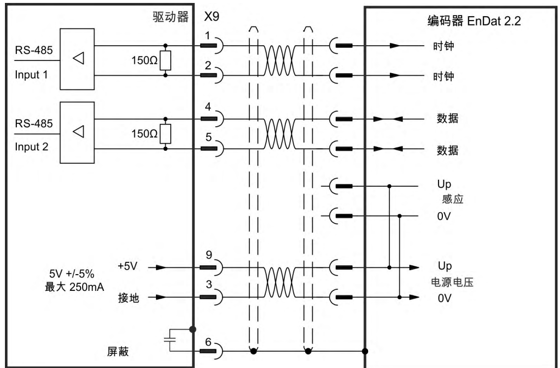
连接图
