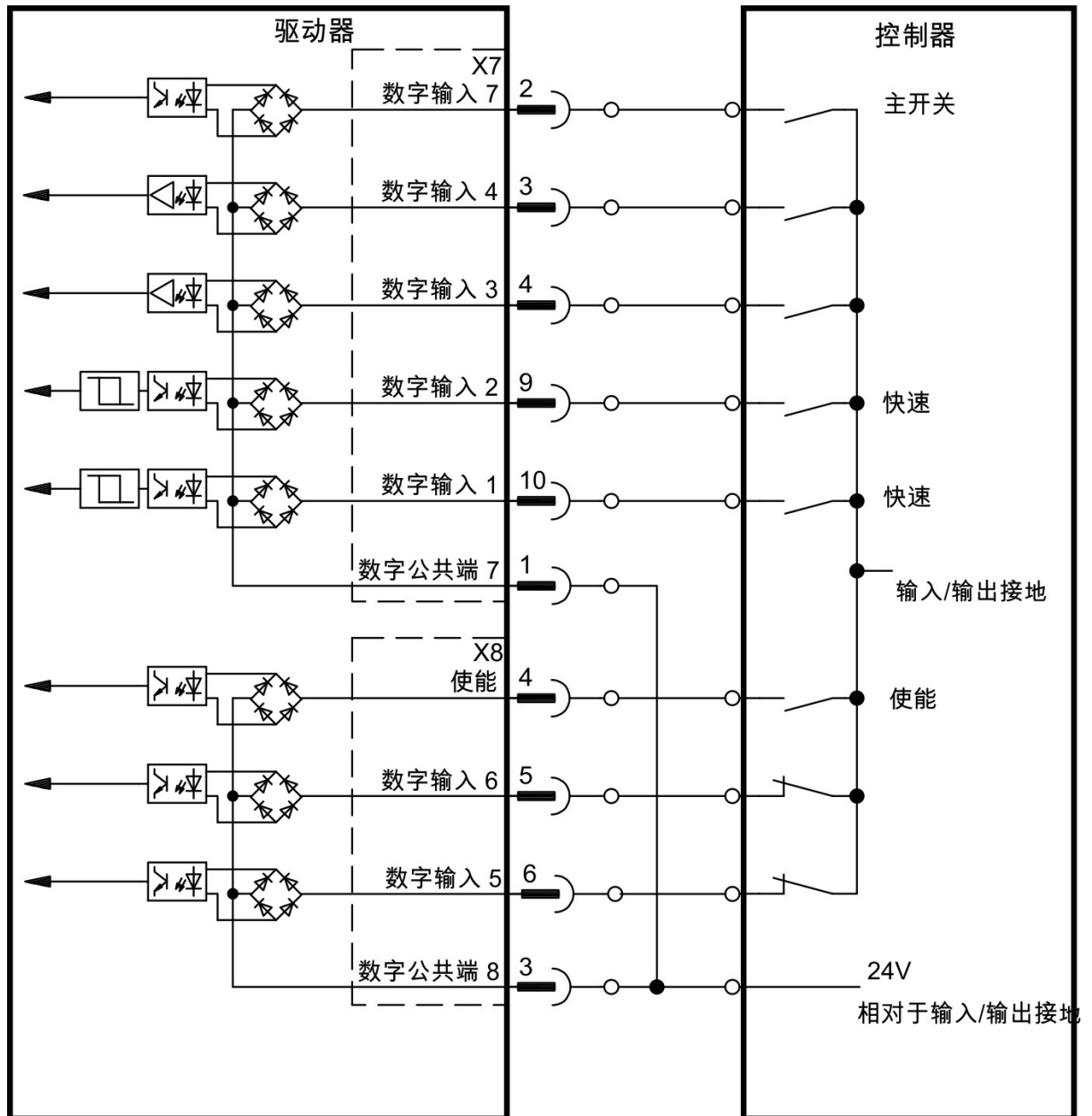
数字输入接线图 X7/X8 (例如, 漏类型连接)
