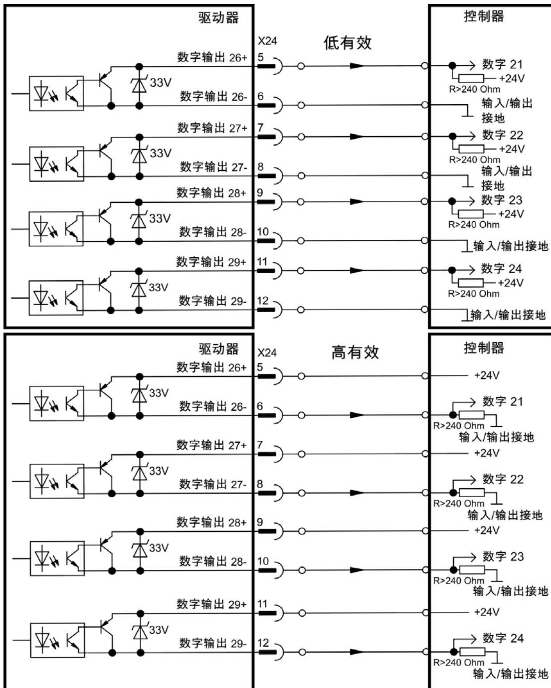
接线图 X24
