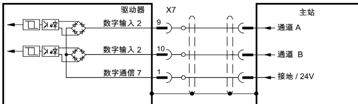
连接图
