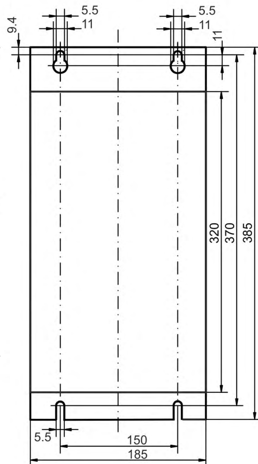
AKD largeur grande 480V, 48A
