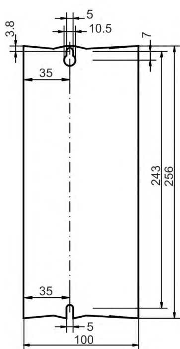
AKD largeur grande 480V, 3A - 12A
