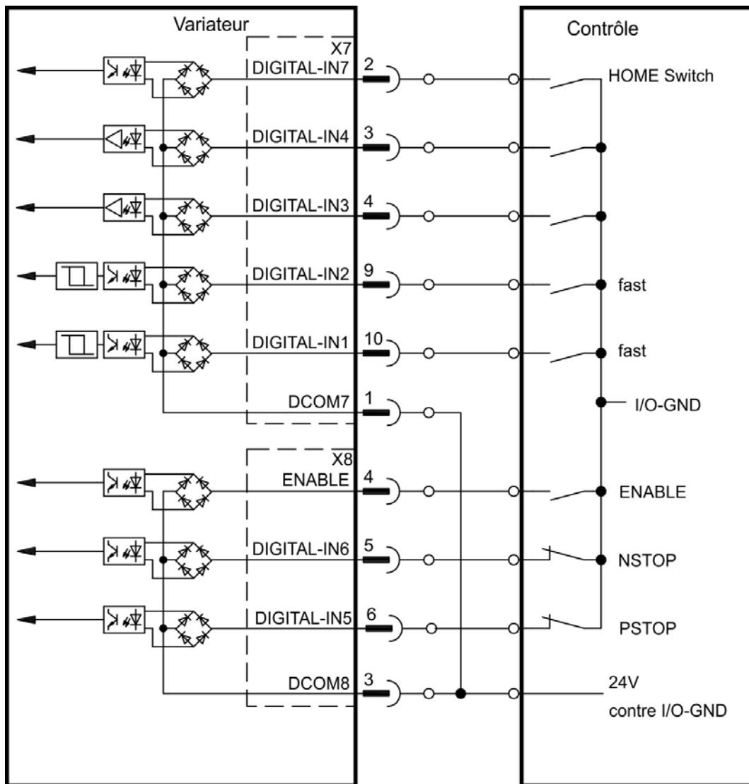
Schéma de raccordement X7/X8 (connexion de type Source, exemple)
