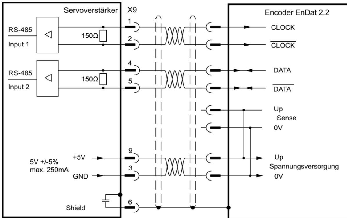
Anschlussbild
