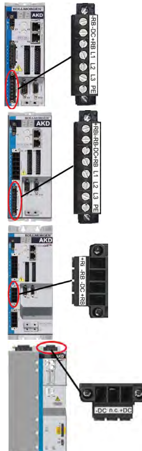
AKD-x00306 bis AKD-x00606 (X3)
