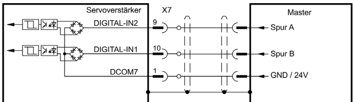
Anschlussbild
