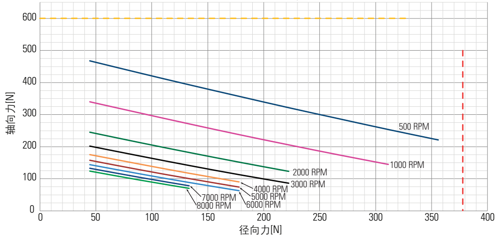
AKM2G-3x电机-20,000小时 L 10 轴承寿命
