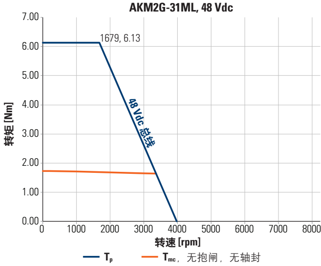
AKM2G-3x转矩-转速性能曲线-最高为96 Vdc电压
