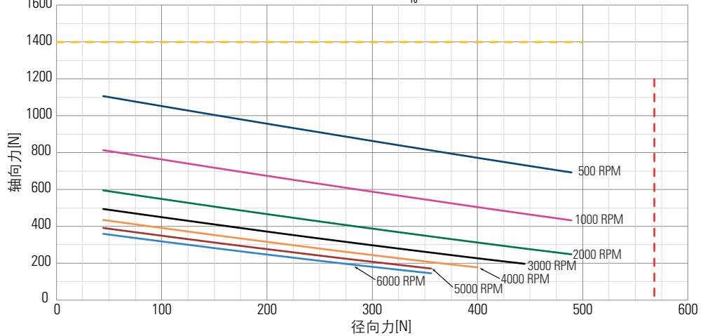
AKM2G-4x电机-20,000小时 L 10 轴承寿命
