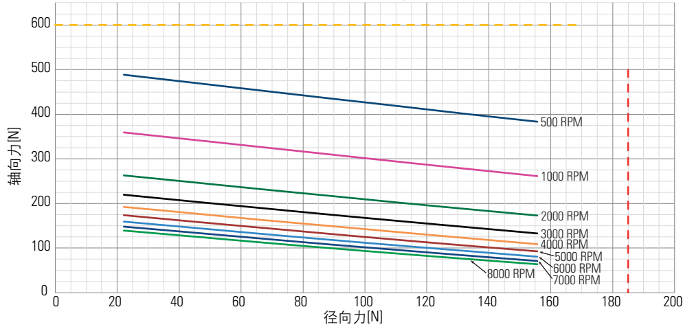
AKM2G-2x电机-20,000小时 L 10 轴承寿命
