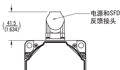
图中给出了“D”连接器选件
