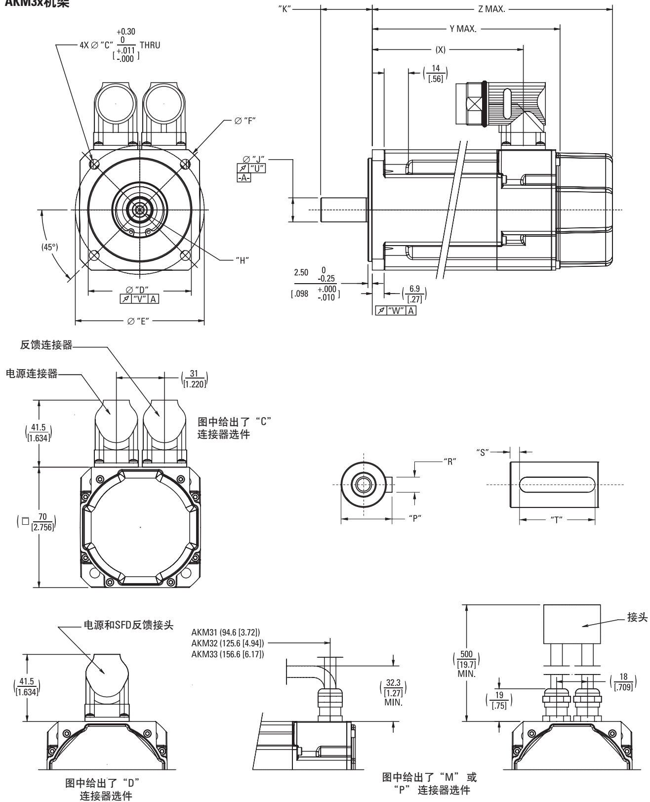
AKM3x机架
