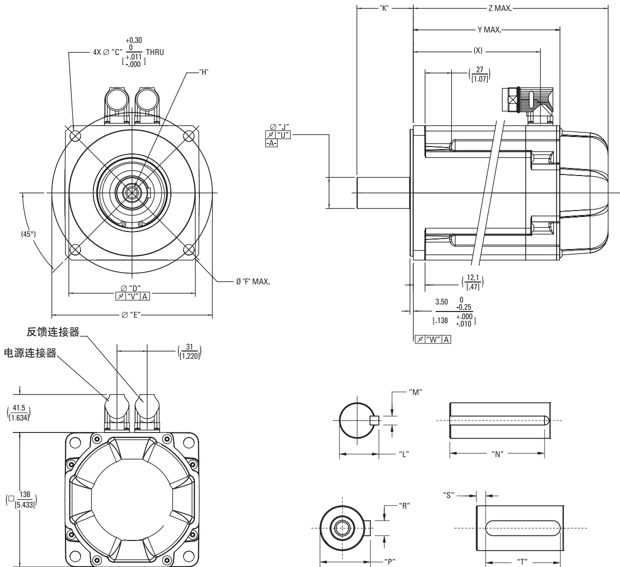
AKM6x机架
