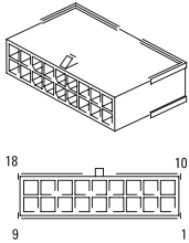
接头部件号: Molex 43020-1801
