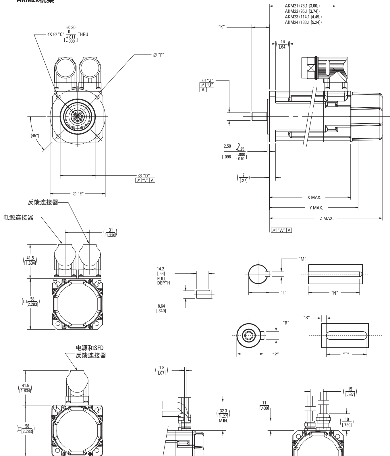
AKM2x机架
