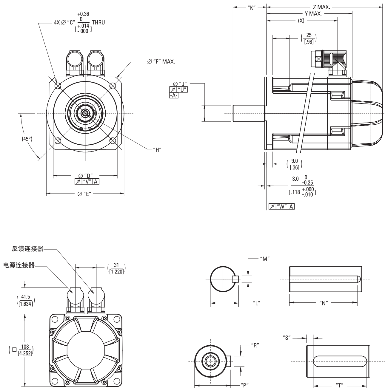
AKM5x机架
