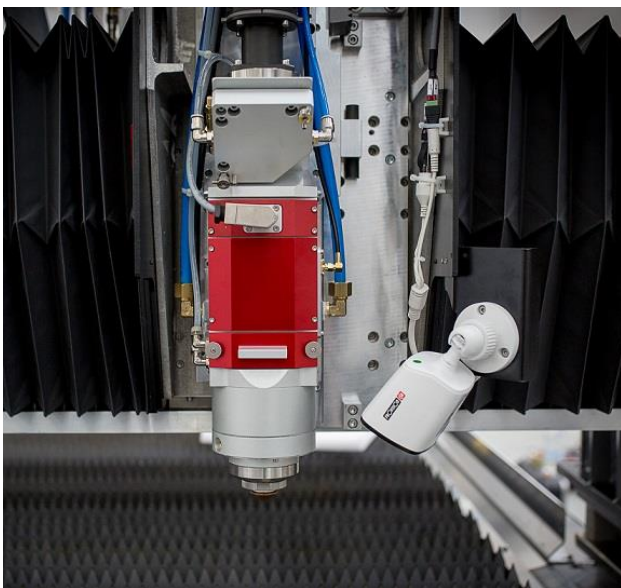
Detail des Laserkopfs Penta Fiber Head by Cutlite Penta und gehäuselose Motoren der Serie KBM von KOLLMORGEN.
