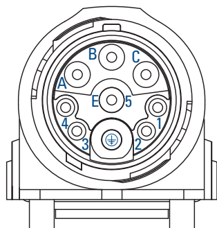
Power + SFD3
